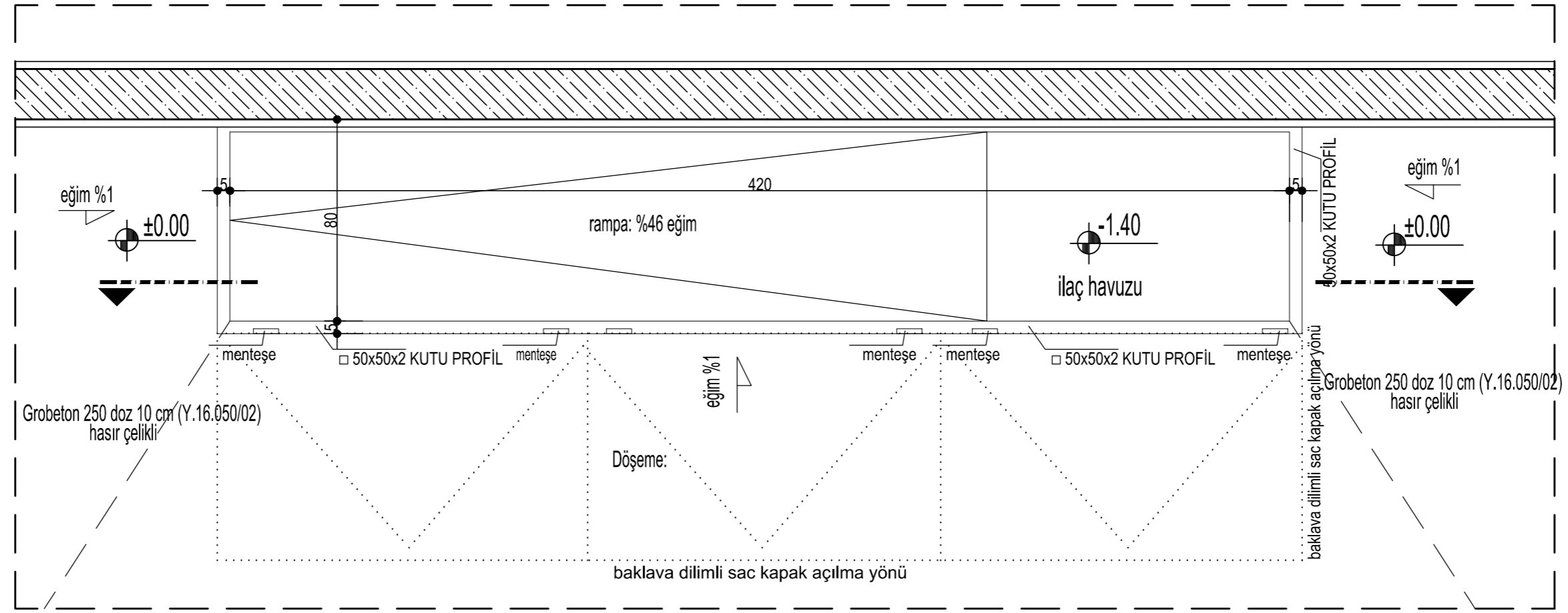
PLAN Ö: 1/20
